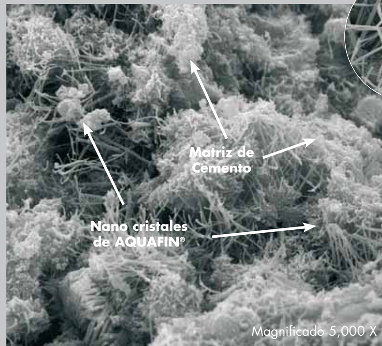
Imagen Magnificada (10,000X) de nano cristales de AQUAFIN®-IC.
